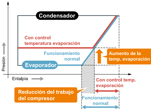
[1] Control de temperatura de evaporación (temperatura fija)
