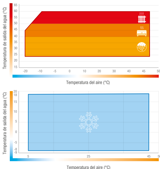
Límites de funcionamiento
