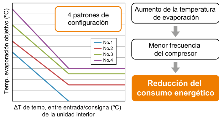
[2] Control de temperatura de evaporación (control automático en 4 patrones)
